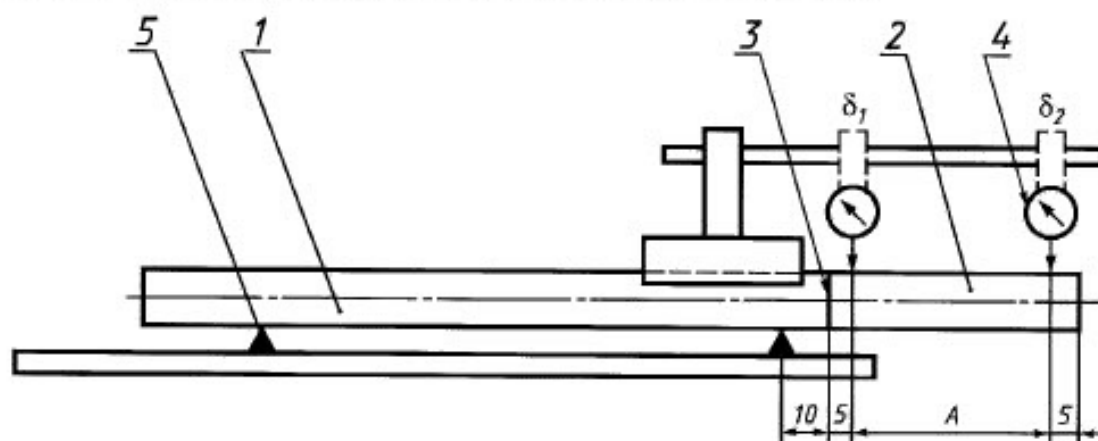
1 — труба; 2 — деталь приварного замка; 3 — сварное соединение (шов); 4 — индикатор часового типа; 5 — ножевая опора; \delta_1, \delta_2 — сечения, в которых измеряют биение; A — расстояние между сечениями
